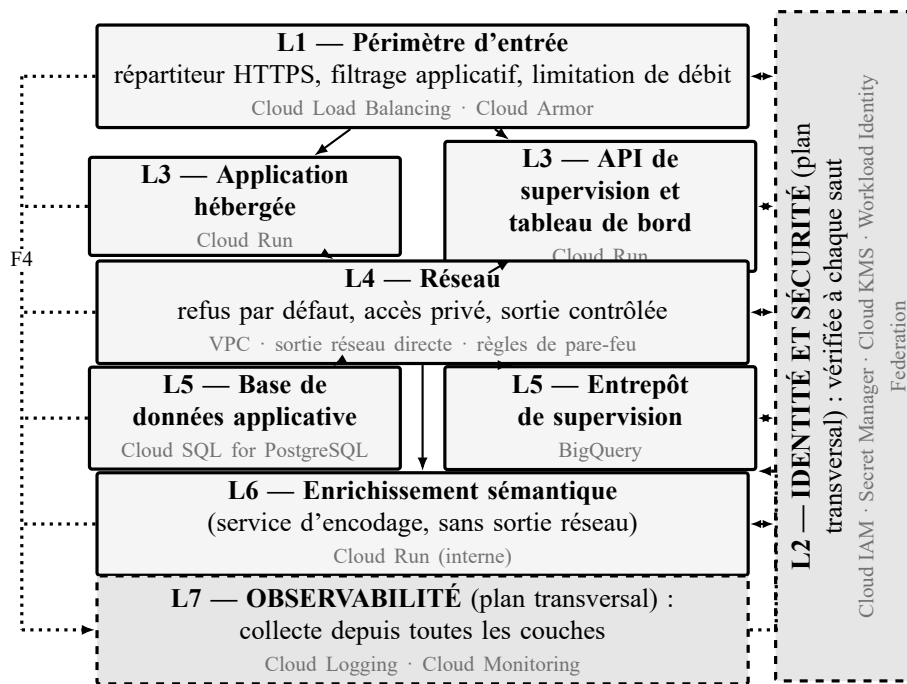
FIG. 9. Modèle en couches : cinq couches empilées (L1, L3, L4, L5, L6) et deux plans transversaux (L2, L7), dont la bordure en tirets marque la portée : L2 vérifie l'identité à chaque saut, L7 collecte depuis toutes les couches. Pointillés : collecte F4. La résolution de noms ne figure pas en L1 : elle est une dépendance externe (figure 8).
