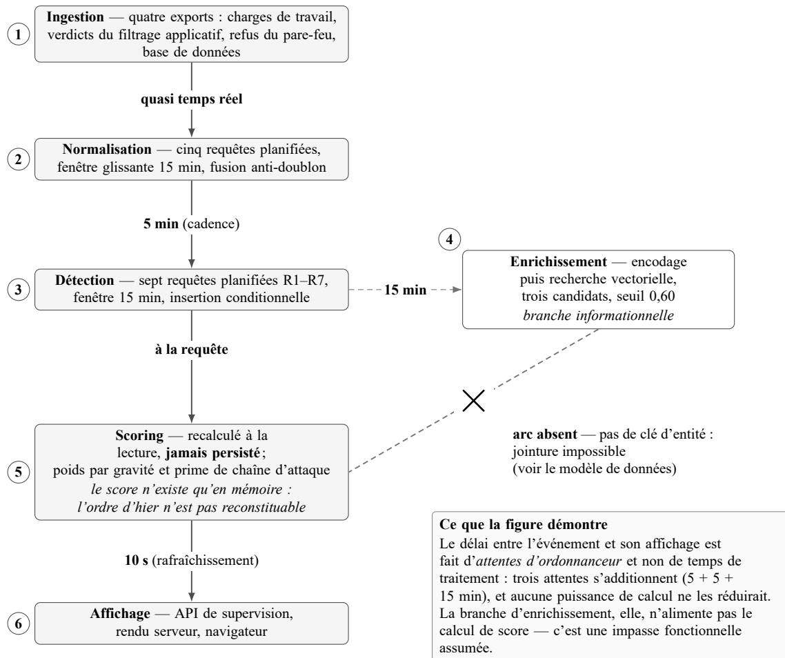
FIG. 13. Cycle de vie de la donnée de sécurité : six étapes, et le budget de latence porté par les cadences
